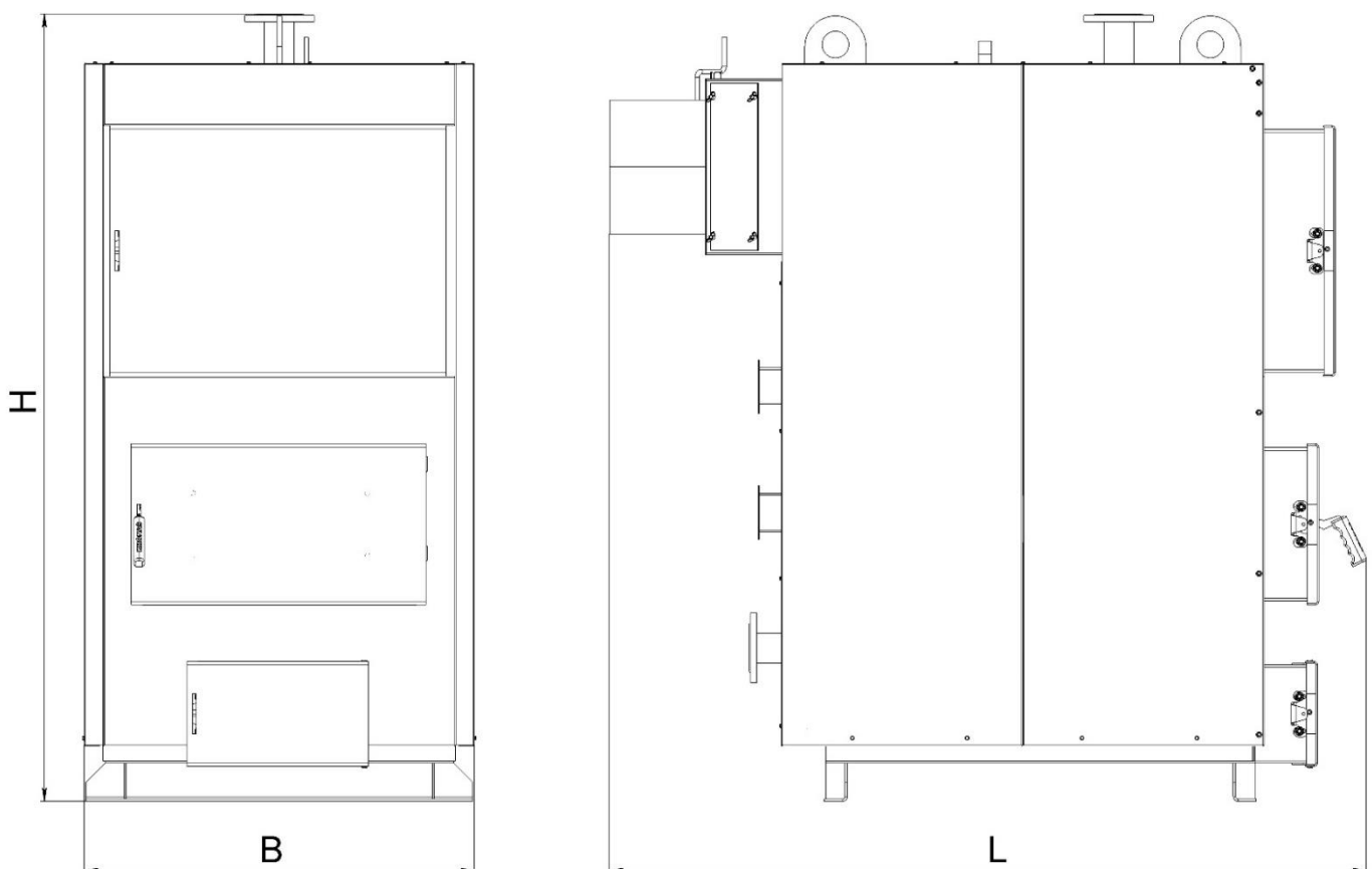
Рисунок 3.1 – Позначення габаритів котла типу КТШ
