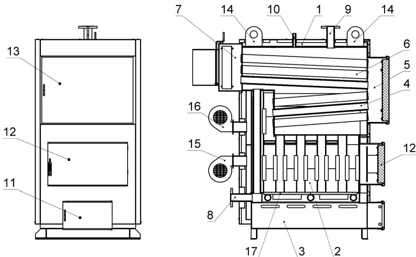
Рисунок 5.1 – Зовнішній вигляд та основні елементи котлів типу КТШ
